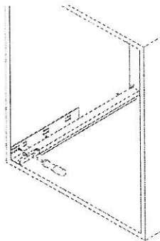
Fissaggio guide laterali (v.foratura pag.2) Fixing lateral slide (see drilling pag.2)
