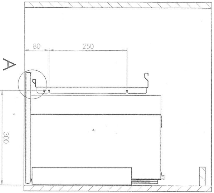
DETTAGLIO A SCALA 2:7
